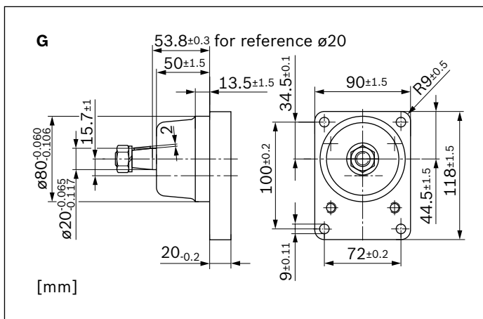
Palier avant Ø80 mm, type 2
