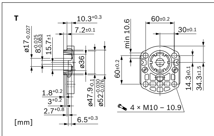
Fixation à 4 trous Ø52 mm, avec joint torique
