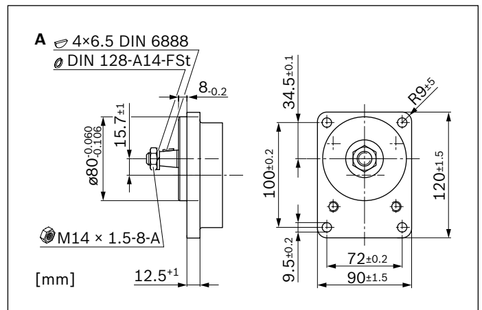
Palier avant Ø80 mm, type 1
