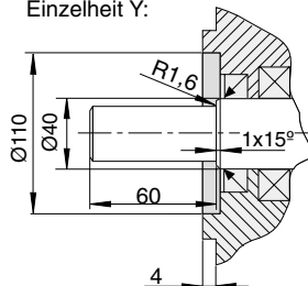
Einzelheit Y:
